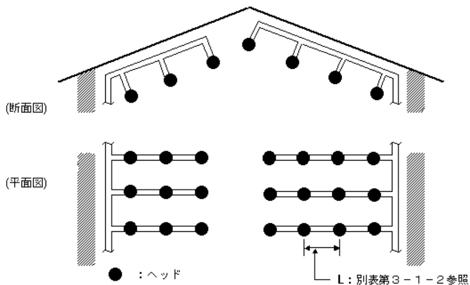
〔正方形又は矩形配置の場合の例〕
