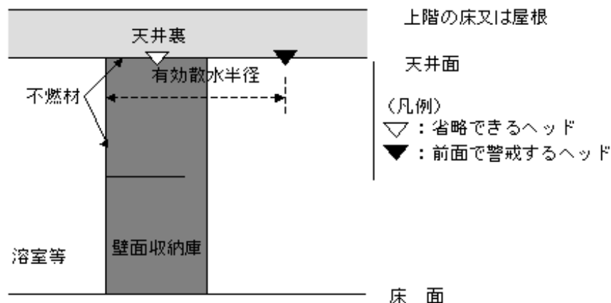
〔壁面収納庫の上部のヘッドを省略した例〕
