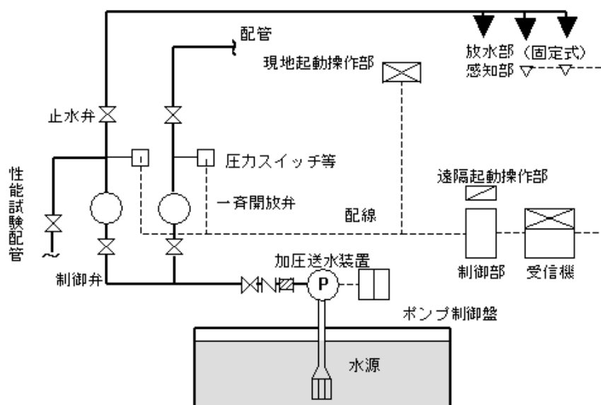
図1 〔放水型スプリンクラー設備(固定式ヘッド)システム系統例〕
