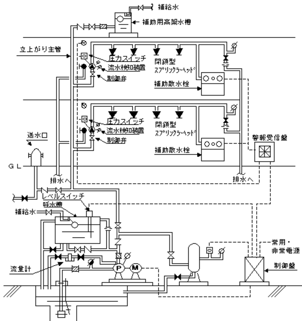
〔閉鎖型スプリンクラー設備の配管系統例〕
