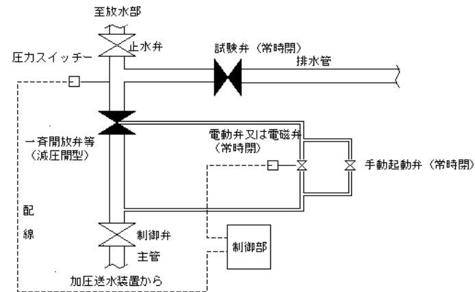
図6 〔加圧方式の一斉開放弁等の廻りの配管図例〕
