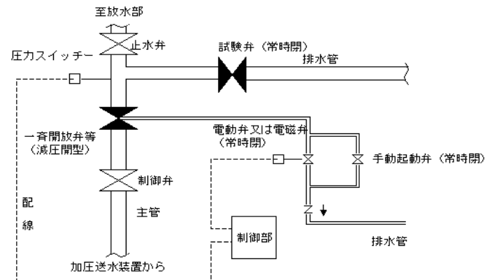
図5 〔減圧方式の一斉開放弁等の廻りの配管図例〕
