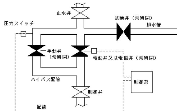
図7 〔電動弁又は電磁弁方式の廻りの配管図例〕
