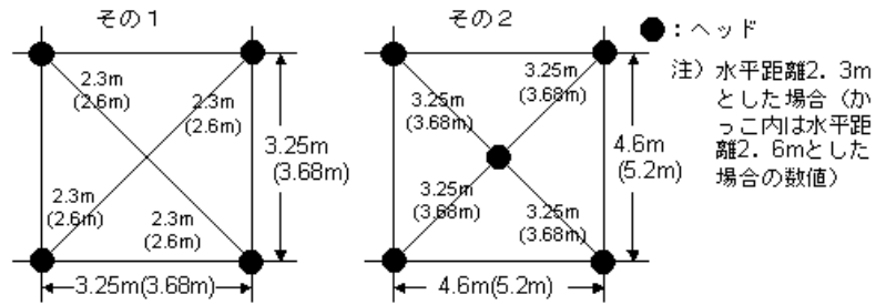
〔格子配列の例〕
