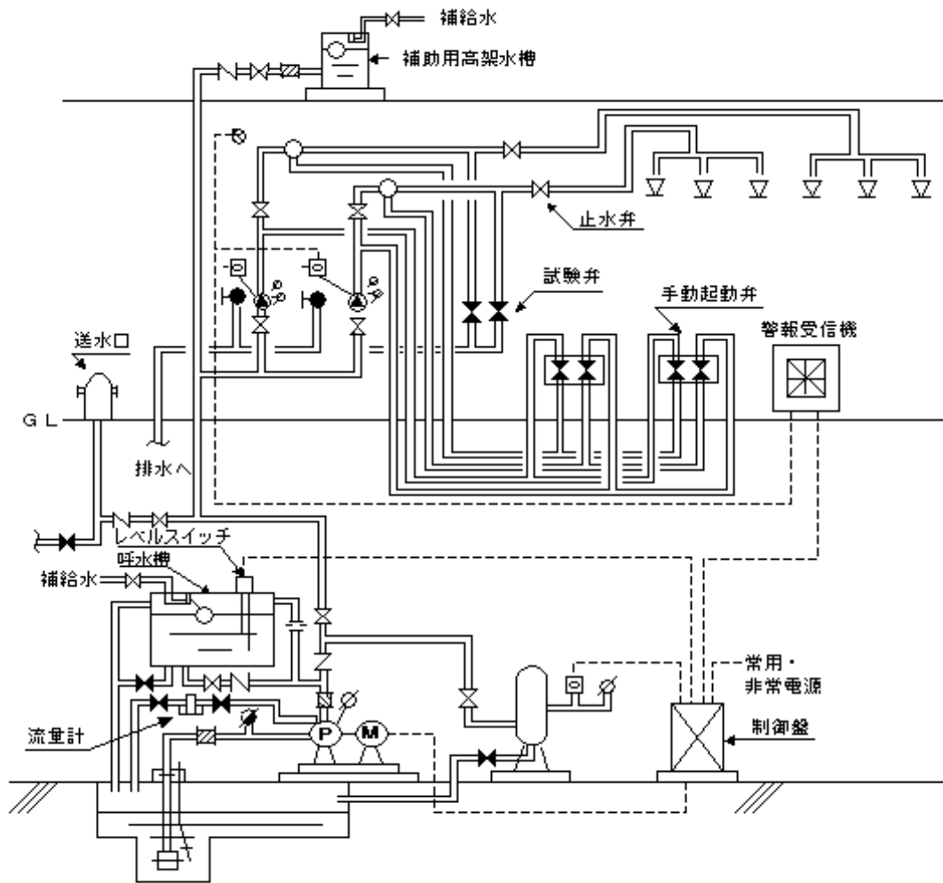
〔開放型スプリンクラー設備の配管系統例〕
