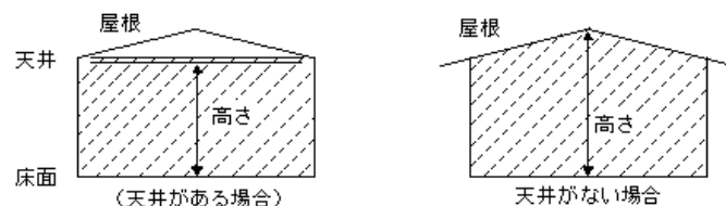
〔床面から天井までの高さの例〕
