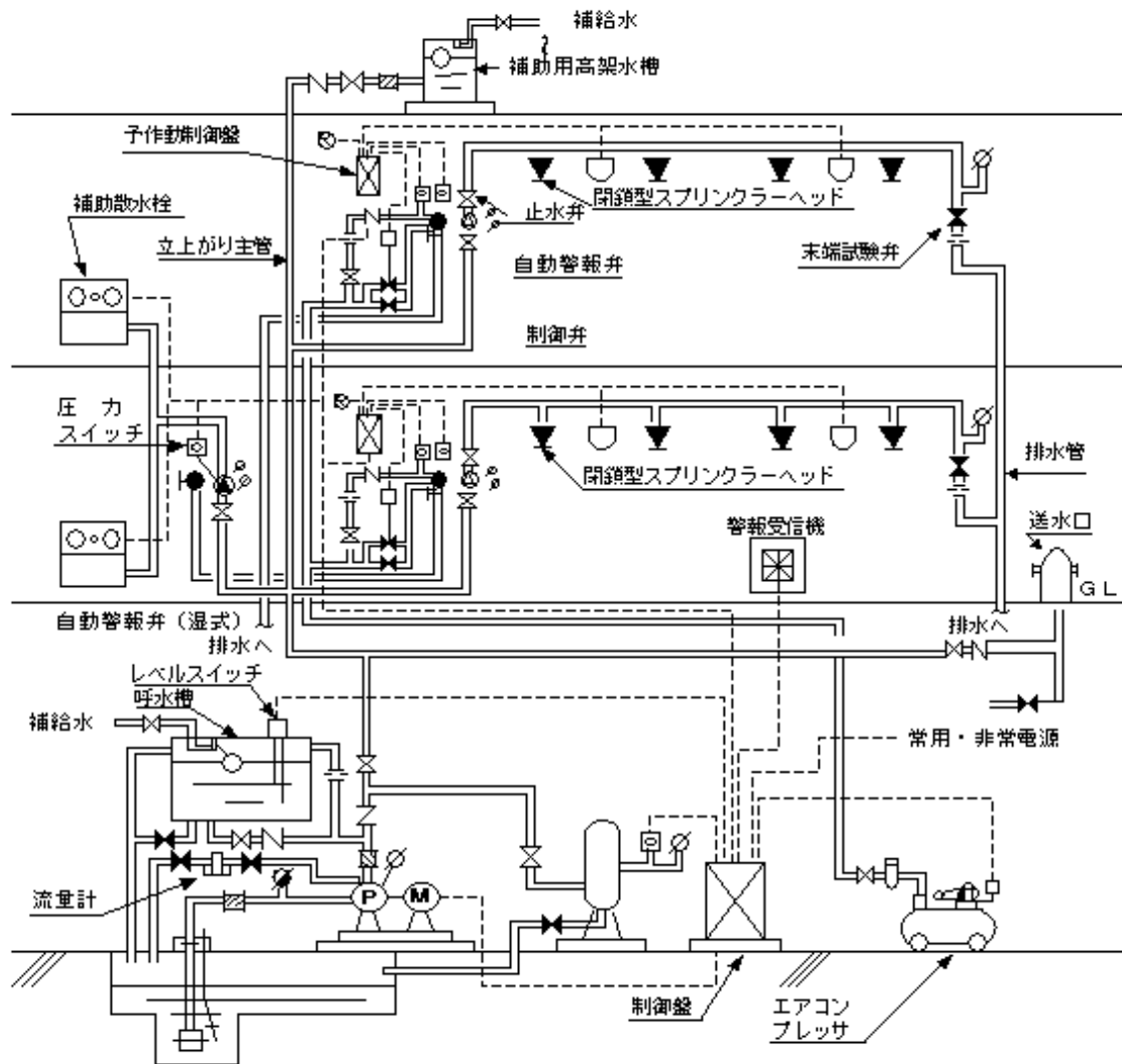
〔予作動式スプリンクラー設備の配管系統例〕
