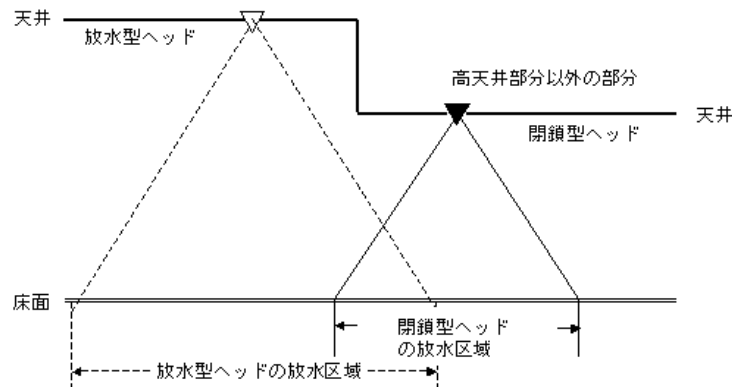
図4 〔放水区域等が重複する設置例〕
