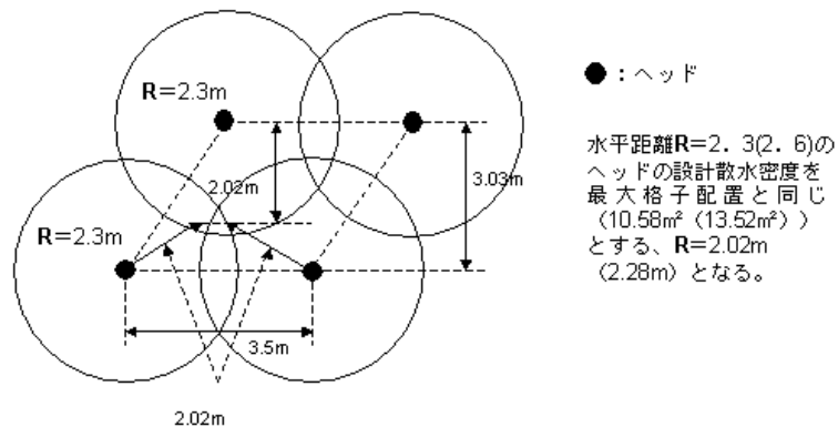
〔散水密度が低下しないようにした千鳥型配置の例〕
