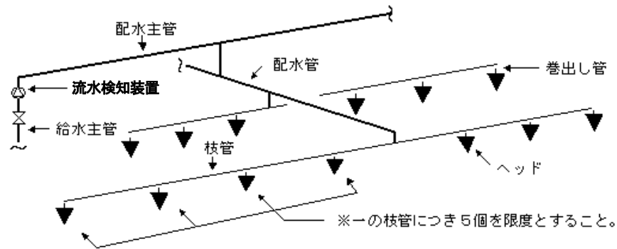
〔配管の名称及び枝管とヘッドの取付け例〕
