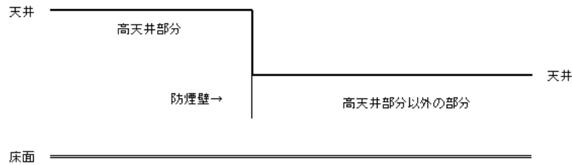
図3 〔防煙壁等の設置例〕
